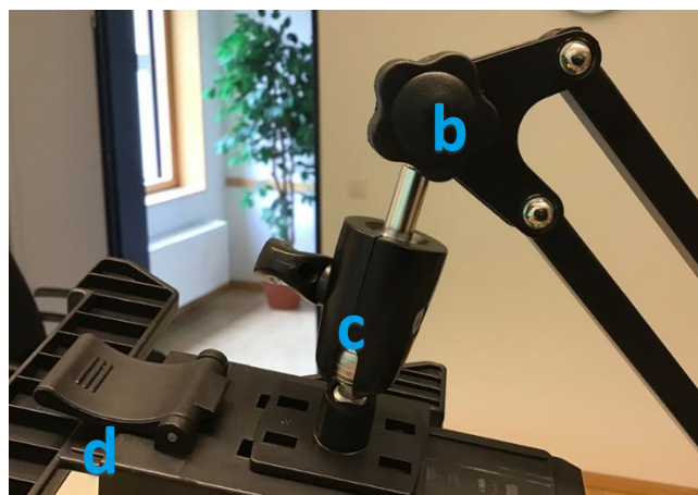
Aufbau Stativ Schwenkarm
